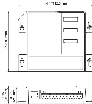
Power Module
